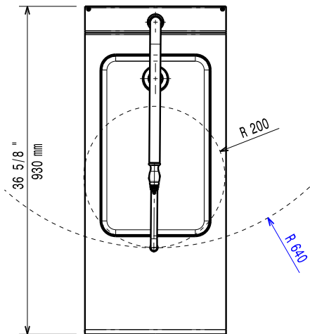
Boven aanzicht
