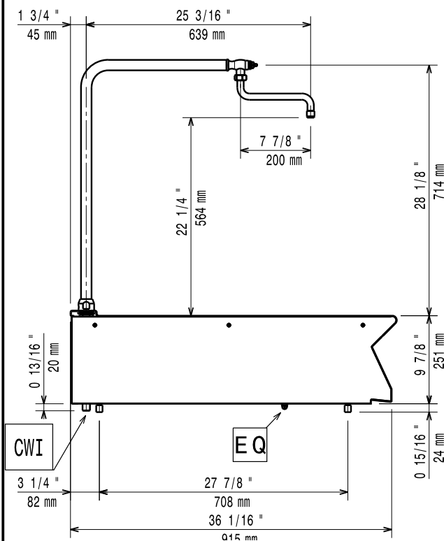
Zij aanzicht
